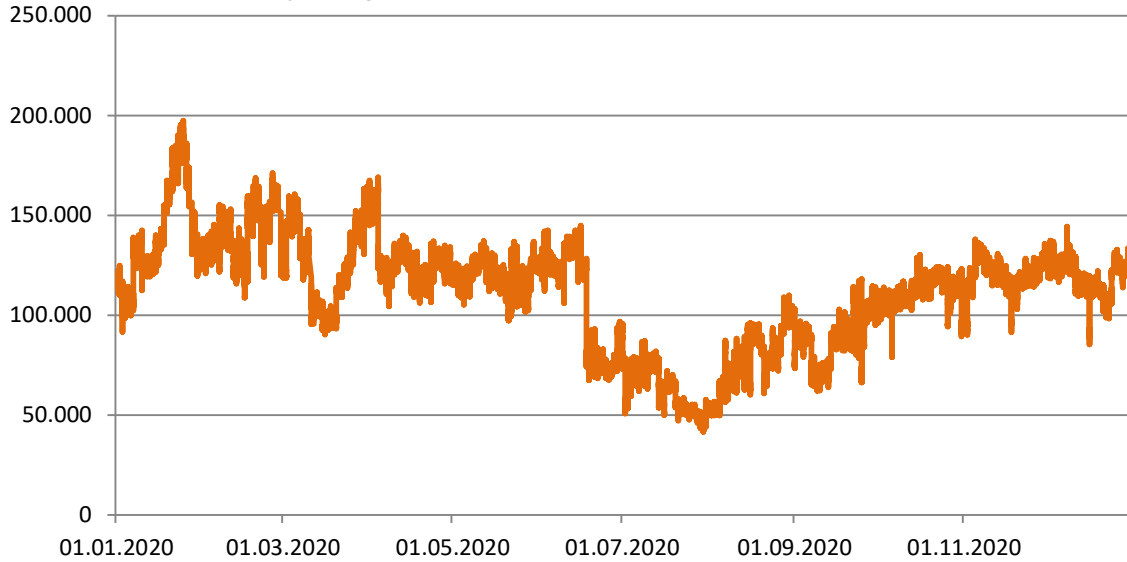
Summe der HS/MS-Einspeisungen im zeitlichen Verlauf [kW]
