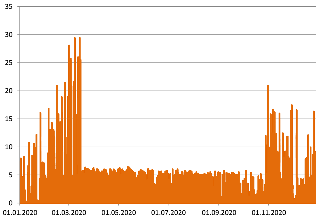
Summe der NS-Einspeisungen im zeitlichen Verlauf [kW]
