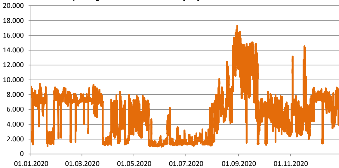
Summe der MS-Einspeisungen im zeitlichen Verlauf [kW]
