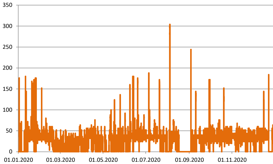
Summe der MS/NS-Einspeisungen im zeitlichen Verlauf [kW]
